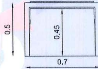
ALZADO FRONTAL
